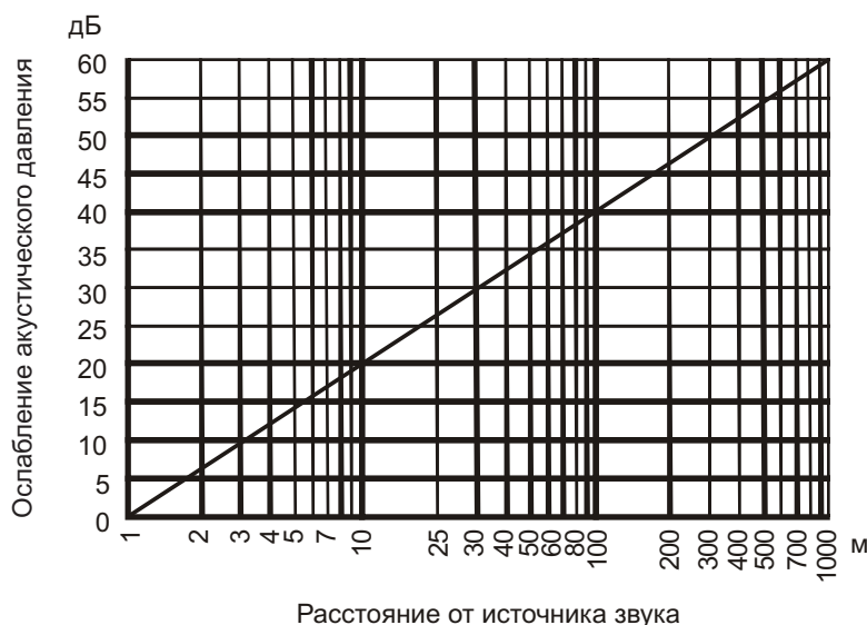
Рисунок С.1 — График зависимости ослабления звукового давления от расстояния до источника звука
